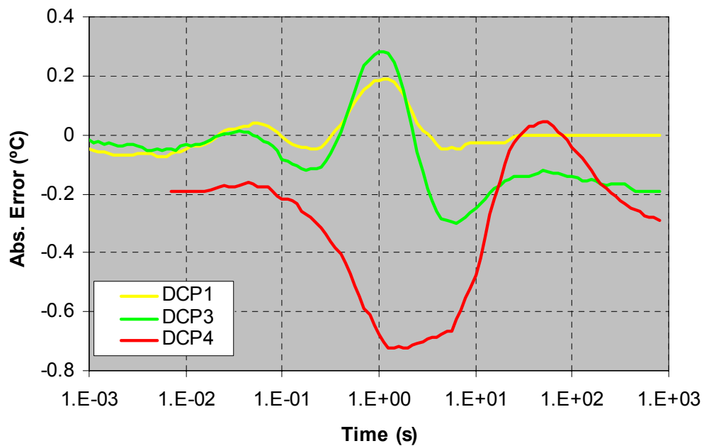
Fig. 4.1: TFBGA 12x12 148 - F.C. – Absolute error
