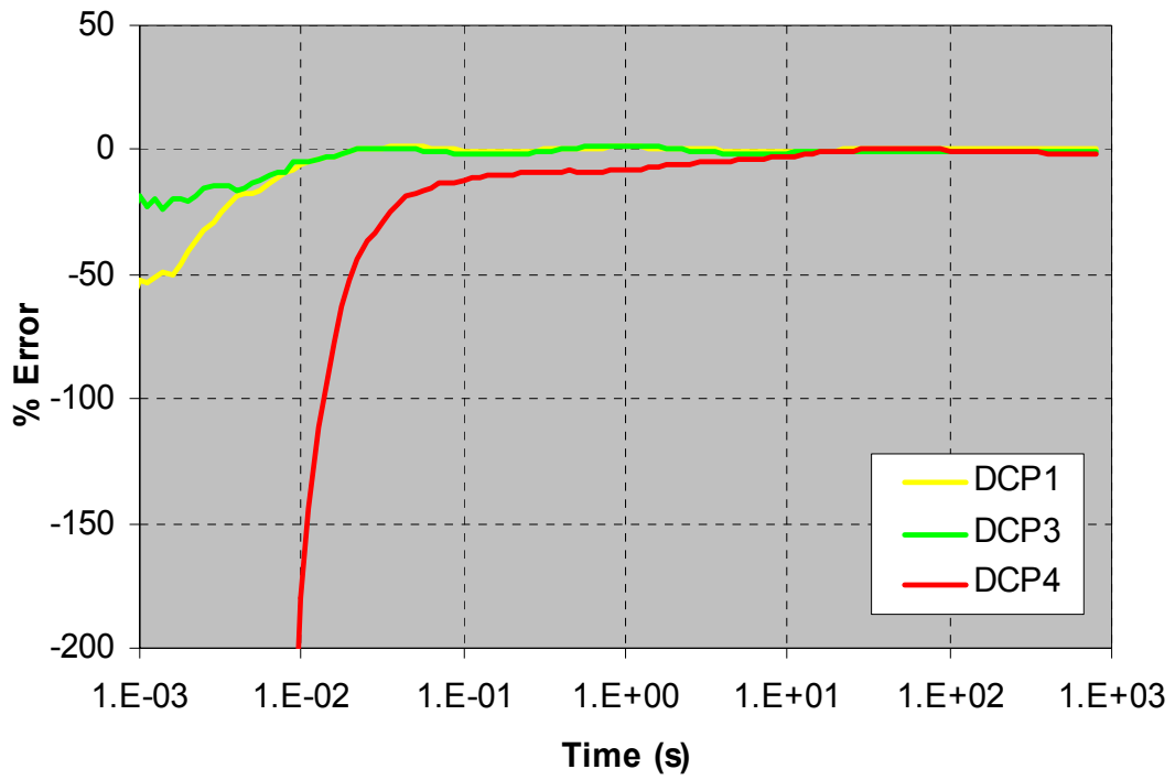
Fig. 4.2: TFBGA 12x12 148 - F.C. – Error (%)
